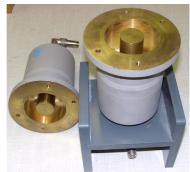
Bild 3 Messanordnung zur Ermittlung der Schirmdämpfung mit TEM-Messköpfen
