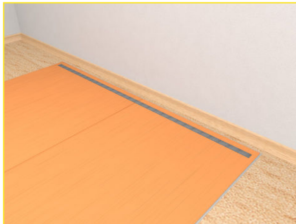
Abb. 23: Erdungsband verkleben (nur bei 2 oder mehr Bahnen)
