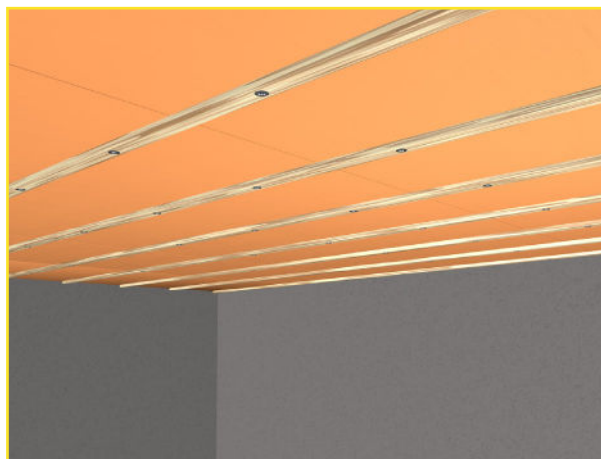
Abb. 19: Fixe Befestigung der Bahnen - Entfernen der Hilfsnägeln
